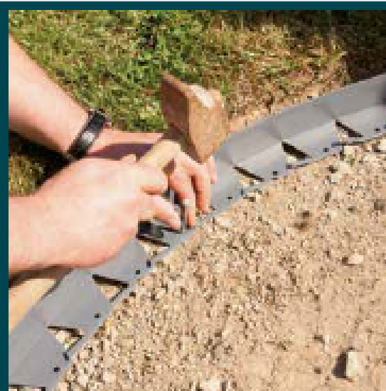
3 Posez le Tcourb'
